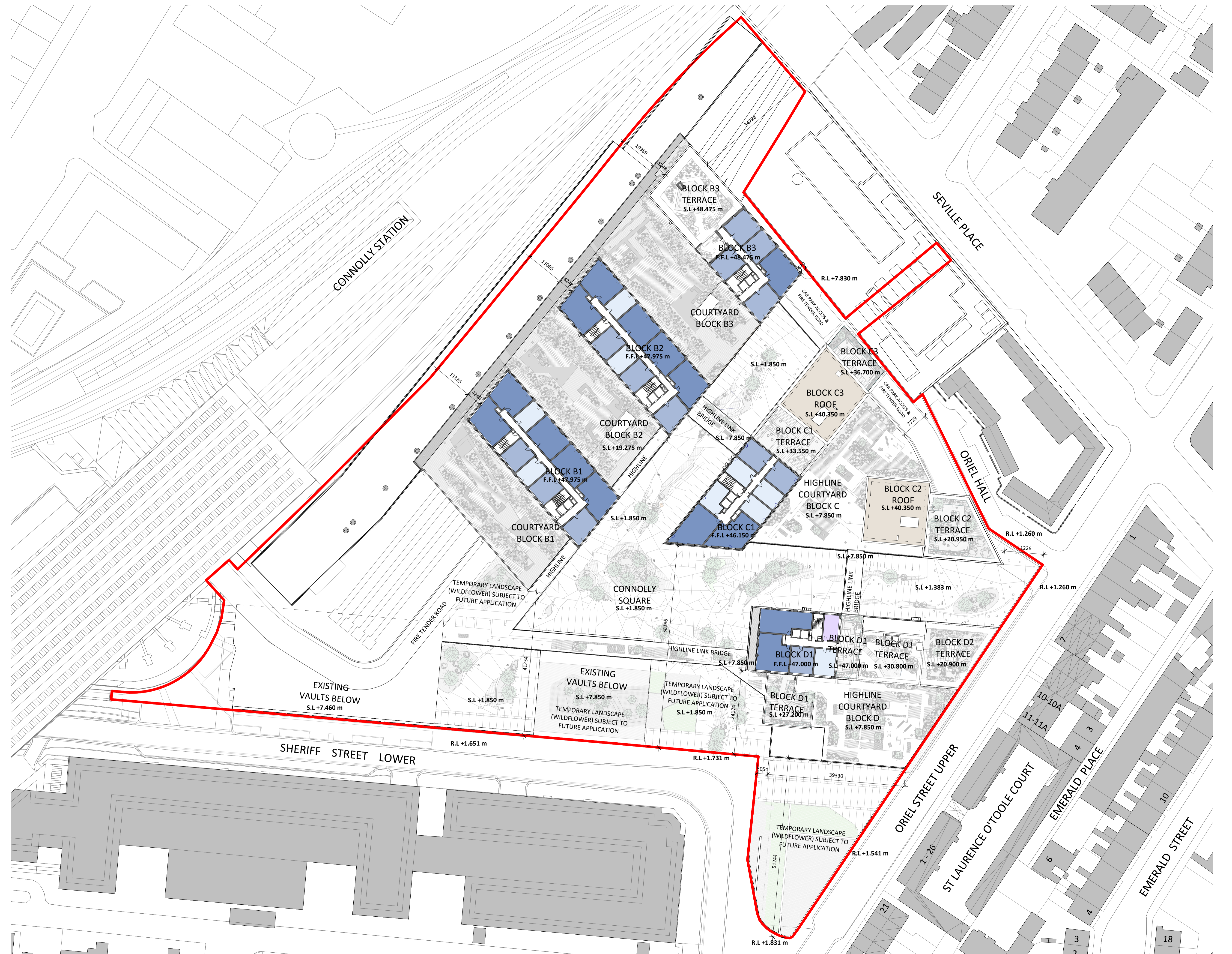
1 SITE LAYOUT PLAN - LEVEL 13 1 : 500
